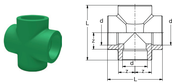
BR PP-RCT Kreuzstück SDR11 grün BR PP-RCT Cross SDR11 green
