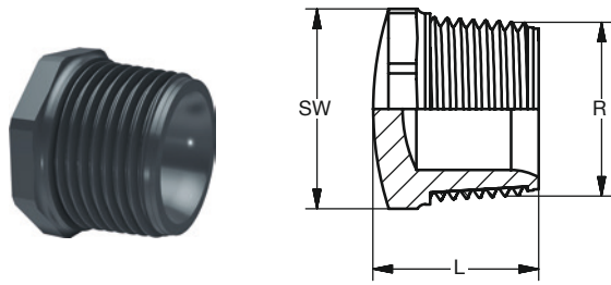
BR PVC-U Stopfen AG-keg grau
