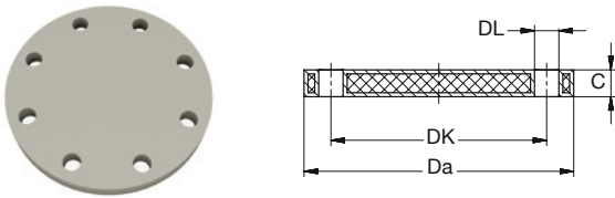
BR PP-St Blindflansch ANSI kieselgrau BR PP-St Flange blind ANSI pebble grey
