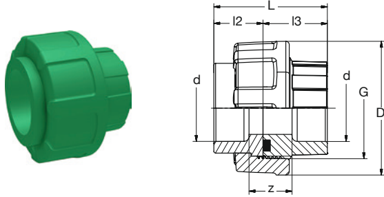
BR PP-RCT Verschraubung Runddichtring-EPDM 20°C/1,0MPa grün BR PP-RCT Union O-Ring-gasket-EPDM 20°C/1.0MPa green
