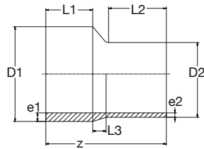
BR PE100 Reduktion kurz exzentrisch SDR17 schwarz BR PE100 Reducer short excentric SDR17 black
