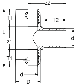
BR PE100 E-T-Stück 90° mit Schweißstutzen SDR11 schwarz BR PE100 E-Tee 90° with spigot SDR11 black
