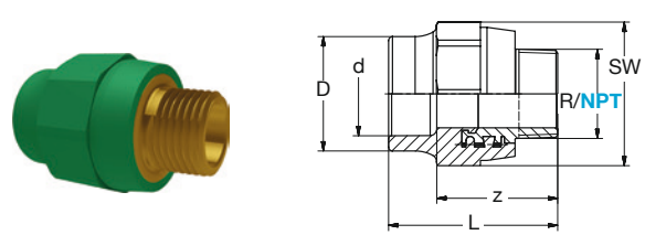
BR PP-RCT-LFB Übergang AG-keg grün
