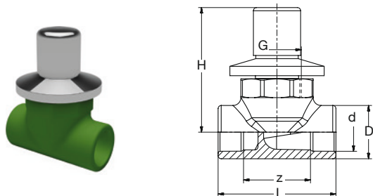
BR PP-R-Ms Ventil Geradsitz UP mit Flügelrad + Kappe grün BR PP-R-Brass Valve straight concealed winged wheel + cap green
