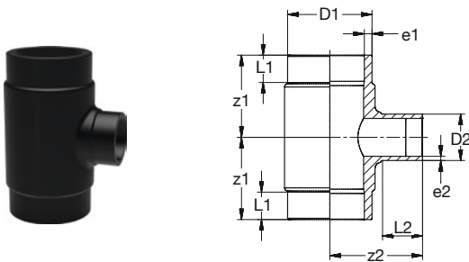
BR PE100 T-Stück 90° red kurz SDR11 schwarz BR PE100 Tee 90° red short SDR11 black
