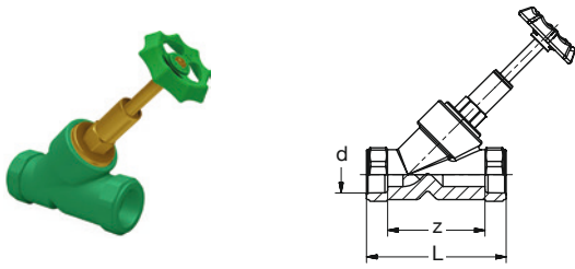
BR PP-RCT Ms-Ventil Schrägsitz mit Metallsitz grün BR PP-RCT Brass-Valve angle with metal seat green
