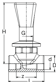
BR PP-RCT-Ms Ventil Geradsitz UP mit Drehgriff grün BR PP-RCT-Brass Valve straight concealed with handle bar green
