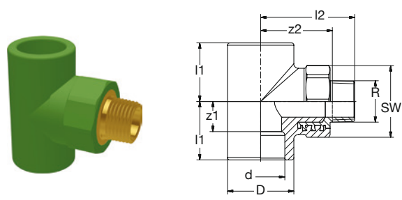
BR PP-R-RG/LFB Ü-T-Stück 90° AG-keg grün
