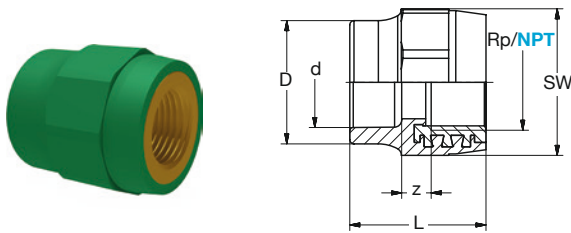
BR PP-RCT-RG/LFB Übergang IG-zyl grün
