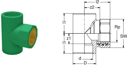
BR PP-RCT-RG/LFB Ü-T-Stück 90° IG-zyl grün
