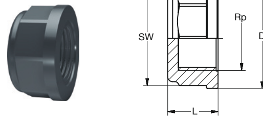
BR PVC-U Kappe IG-zyl grau
