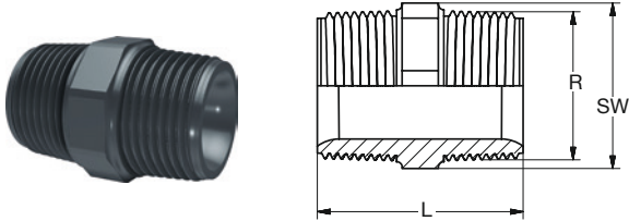
BR PVC-U Doppelnippel AG-keg grau
