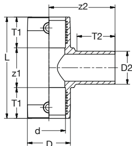
BR PE100 E-T-Stück 90° red mit Schweißstutzen SDR11 schwarz BR PE100 E-Tee 90° red. with spigot SDR11 black
