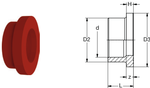
BR PP-CFR Bundbuchse rot
