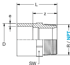
BR PE100 Übergang kurz AG-keg SDR11 schwarz BR PE100 Transition short male-thread-con SDR11 black
