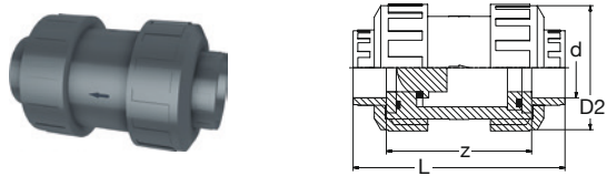
BR PVC-U Ventil Rückschlag Runddichtring-EPDM grau BR PVC-U Valve non-return O-Ring-gasket-EPDM grey
