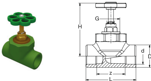
BR PP-R-Ms Ventil Geradsitz mit Handrad grün BR PP-R-Brass Valve straight concealed with hand wheel green
