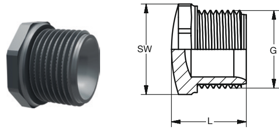
BR PVC-U Stopfen AG-zyl grau
