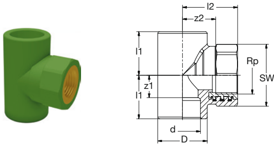
BR PP-R-RG/LFB Ü-T-Stück 90° IG-zyl grün
