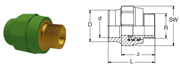
BR PP-R-LFB Übergang AG-keg grün
