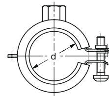
Rohrschelle STANDARD mit Gummieinlage schwarz
