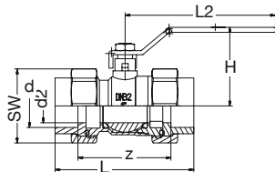
BR PP-RCT Kugelhahn-Ms verschraubt Runddichtring-EPDM 20°C/1,0MPa grün BR PP-RCT Ball valve Brass with union-nuts O-Ring-gasket-EPDM 20°C/1.0MPa green
