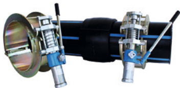
HST Rundungsschelle RSH, Stahl, Oberfläche verzinkt, ohne Hydraulikzylinder HST Rounding clamp RSH, steel, surface galvanized, without hydraulic cylinder
