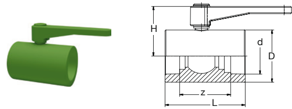
BR PP-R Kugelhahn 20°C/1,0MPa grün BR PP-R Ball valve 20°C/1,0MPa green
