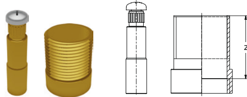
BR Ventil Geradsitz UP Verlängerungsset 25mm
