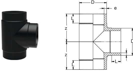
BR PE100 T-Stück 90° kurz SDR11 schwarz BR PE100 Tee 90° short SDR11 black
