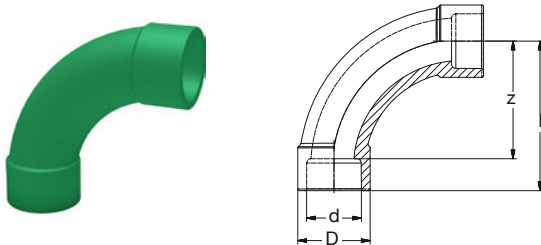
BR PP-RCT Bogen 90° SDR11 grün
