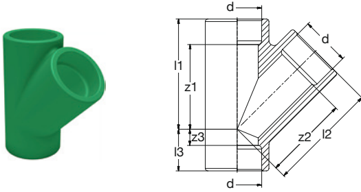
BR PP-RCT Abzweig 45° SDR11 grün BR PP-RCT Branch 45° SDR11 green
