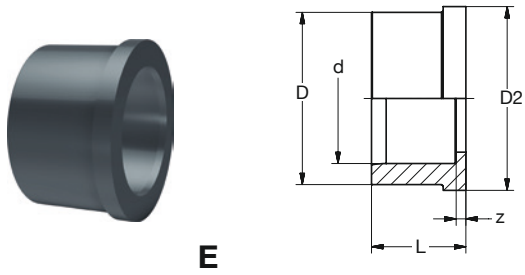
BR PVC-U Verschraubung Einlegeteil grau BR PVC-U Union Insert-part grey
