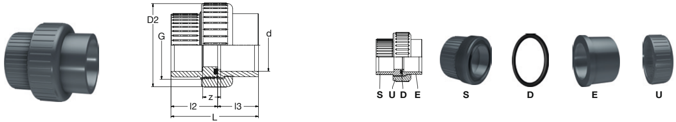
BR PVC-U Verschraubung Runddichtring-EPDM grau BR PVC-U Union O-Ring-gasket-EPDM grey
