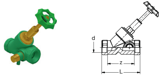
BR PP-RCT Ms-Ventil Schrägsitz mit Metallsitz + Entleerung + Prüfstopfen grün BR PP-RCT Brass-Valve angle with metal seat + drainage + test plug green
