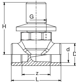
BR PP-RCT-Ms Ventil Geradsitz UP mit Flügelrad + Kappe grün BR PP-RCT-Brass Valve straight concealed with winged wheel + cap green
