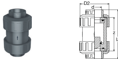
BR PVC-U Ventil Fuß Runddichtring-EPDM grau BR PVC-U Valve foot O-Ring-gasket-EPDM grey
