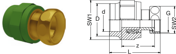
BR PP-R- RG/LFB Anschlussverschraubung für Armaturen + Wasserzähler IG-zy1 mit Flachdichtring-EPDM grün BR PP-R- Bronze/LFB Union flat- sealing for Valves + Water meters female-thread-cyl with flat-gasket-EPDM green
