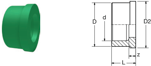
BR PP-RCT Verschraubung Einlegteil grün BR PP-RCT Union Insert-part green
