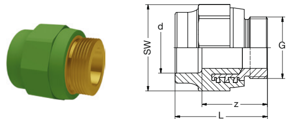
BR PP-R- RG/LFB Verschraubung Schraubteil flachdichtend grün BR PP-R- Bronze/LFB Union Srew-part flat-sealing green
