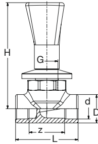
BR PP-R-Ms Ventil Geradsitz UP Drehgriff grün
