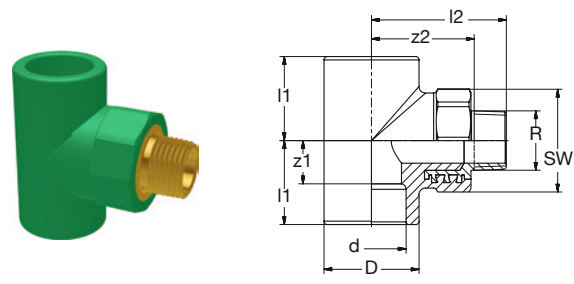
BR PP-RCT-RG/LFB Ü-T-Stück 90° AG-keg grün
