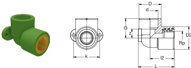
BR PP-R-RG/LFB Ü-Winkel 90° Wandbefestigung IG-zyl grün
