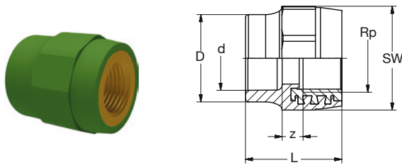
BR PP-R-RG/LFB Übergang IG-zyl grün
